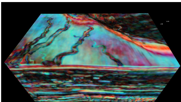
Figura 11 - Método Uniform Constant Q usando as frequências 20Hz (R), 40Hz (G) e 60Hz (B)
