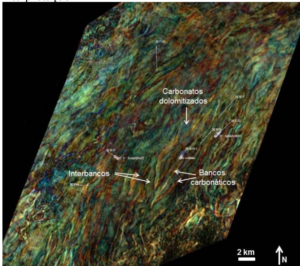
Figura 17 – decomposição espectral no esquema RGB projetado no horizonte topo dos carbonatos marinhos.
