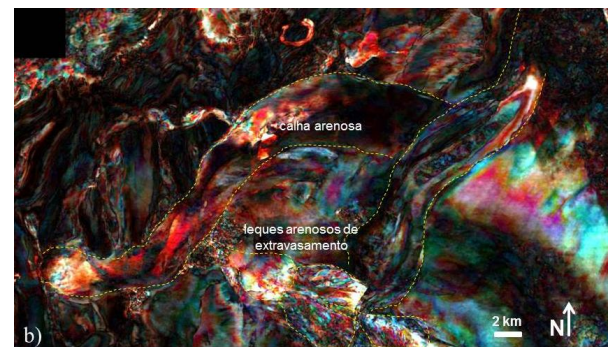
Figura 13 – a) Slice comparando amplitude sísmica com b) colour blend .
