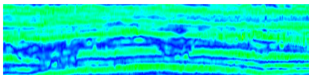
Figura 8 - Método Matching Pursuit - Envelope correspondente a 40 Hz
