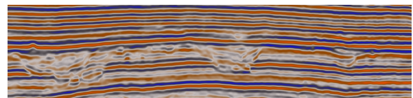
Figura 5 - Série de refletividade (dado de entrada)
